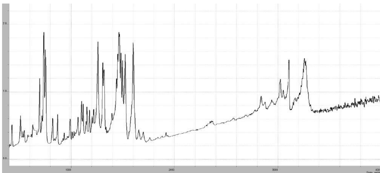
Рис. 1. ИК-спектр 3-фениламинометилтиазоло[3,2-а]бензимидазола (1).
